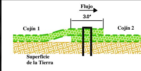
Figura C - Corte de Vista Transversal
