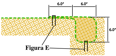
Figura G - Puntos Críticos
