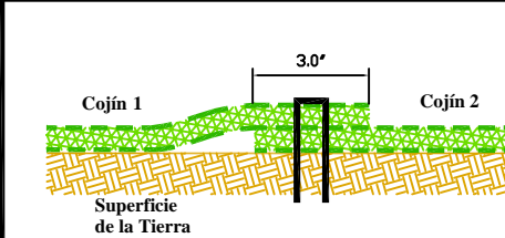
Figura C - Corte de Vista Transversal
