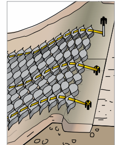
ATRA® Anchors
